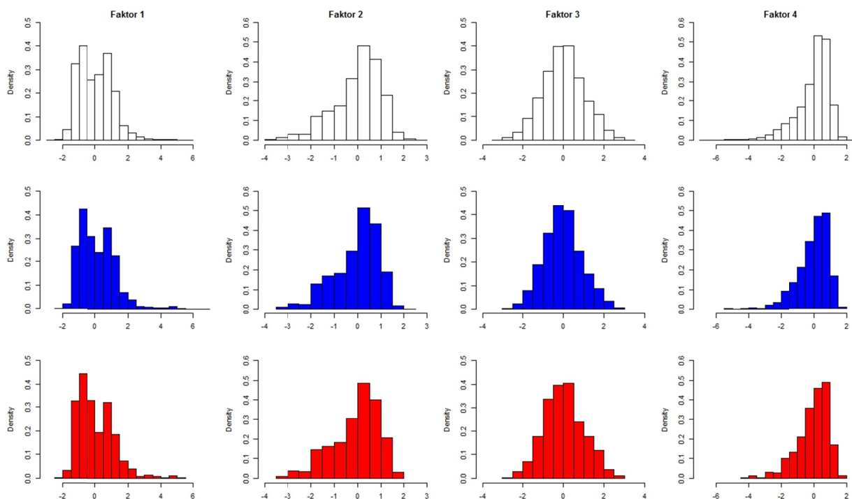
Abb. 4: Datenverteilung der Faktoren (Faktor 1 bis Faktor 4) für die nationale Ebene ( n=344.964 Rasterzellen, obere Zeile), die Länderstichprobe (2637 Stichprobenflächen, mittlere Zeile) und die Bundestichprobe (1000 Stichprobenflächen, untere Zeile).
