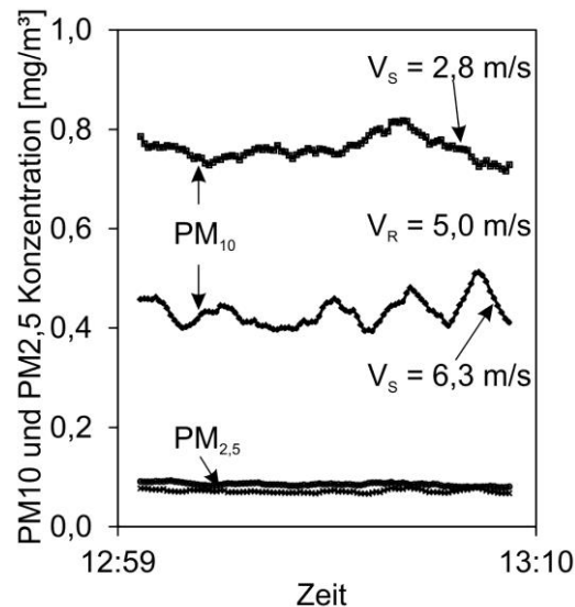
Abb. 3: Gemessene PM 2,5 und PM 10 Konzentrationen in Abhängigkeit vom Geschwindigkeitsverhältnis ( V_s = Sondengeschwindigkeit, V_R = Rohrgeschwindigkeit) (aus Clauß & Hinz 2014)
