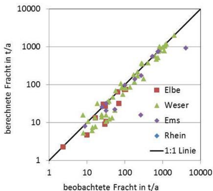
Abbildung 15: Vergleich der beobachteten und berechneten P-Frachten als Gesamtergebnis aus den Modellierungen des AGRUM + -Niedersachsen-Modellverbundes für das Jahr 2007
