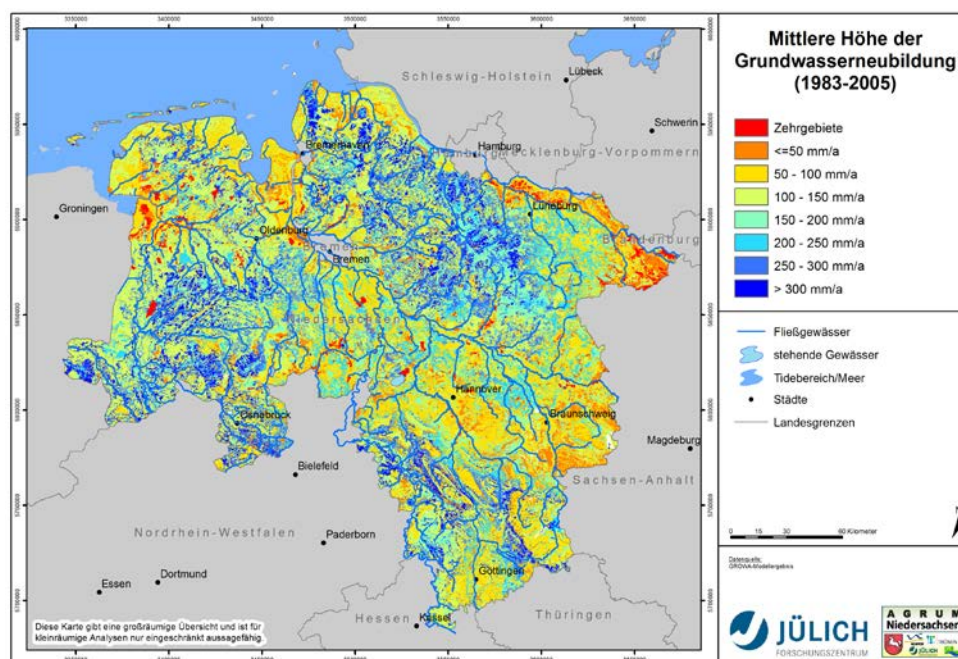
Karte 16: Mittlere jährliche Grundwasserneubildungshöhe (1983 bis 2005) auf Rasterbasis (100 x 100 m)
