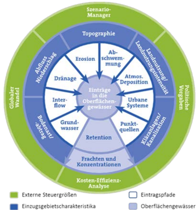
Abbildung 33: Eintragspfade in MONERIS
