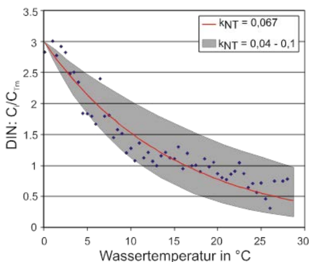
Abbildung 35: Zusammenhang zwischen mittleren C_i/C_{Tm} , berechnet für Temperaturklassen in 0,5° C-Schritten von 0 bis 28° C
