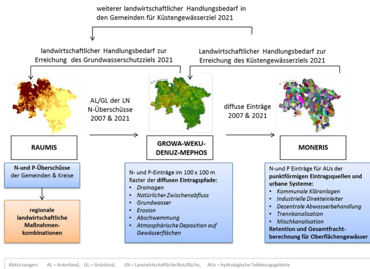
Abbildung 1: Integrativer/Interdisziplinärer Modellverbund
