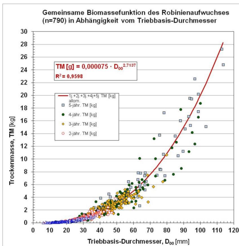
Abb. 2: Allometrische Biomassefunktion über alle FastWOOD II-Modellflächen und Versuchspartzen des ein- bis fünfjährigen Aufwuchses (2009 bis 2013). Als Bezugsgröße dient der Triebbasis-Durchmesser ( d_{00} , mit Rinde in ca. 5 cm Schnitthöhe), da eine Probekreisaufnahme erst nach Flächenräumung möglich ist.
