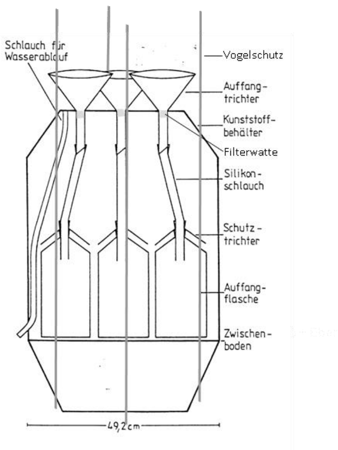
Abbildung 4.5: Bulksammler Typ „Osnabrück“.
