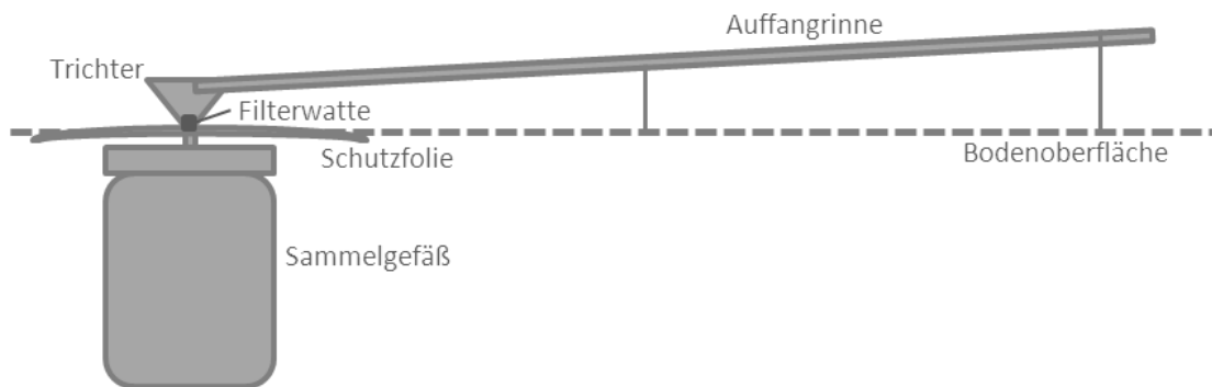
Abbildung 4.8: Aufbau des Rinnen-Messsystems unter Heide.
