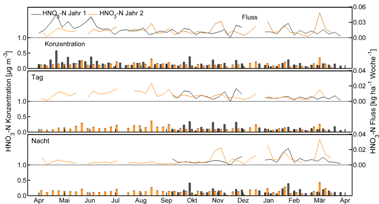
Abbildung 4.14: HNO 3 -Konzentrations- und Depositionsverlauf für beide Messjahre (Jahr 1 = April 2011 bis März 2012, Jahr 2 = April 2012 bis März 2013) am Standort Rühler Moor (oben: gesamt, Mitte: Tageswerte, unten: Nachtwerte; Fehlerbalken = SD).
