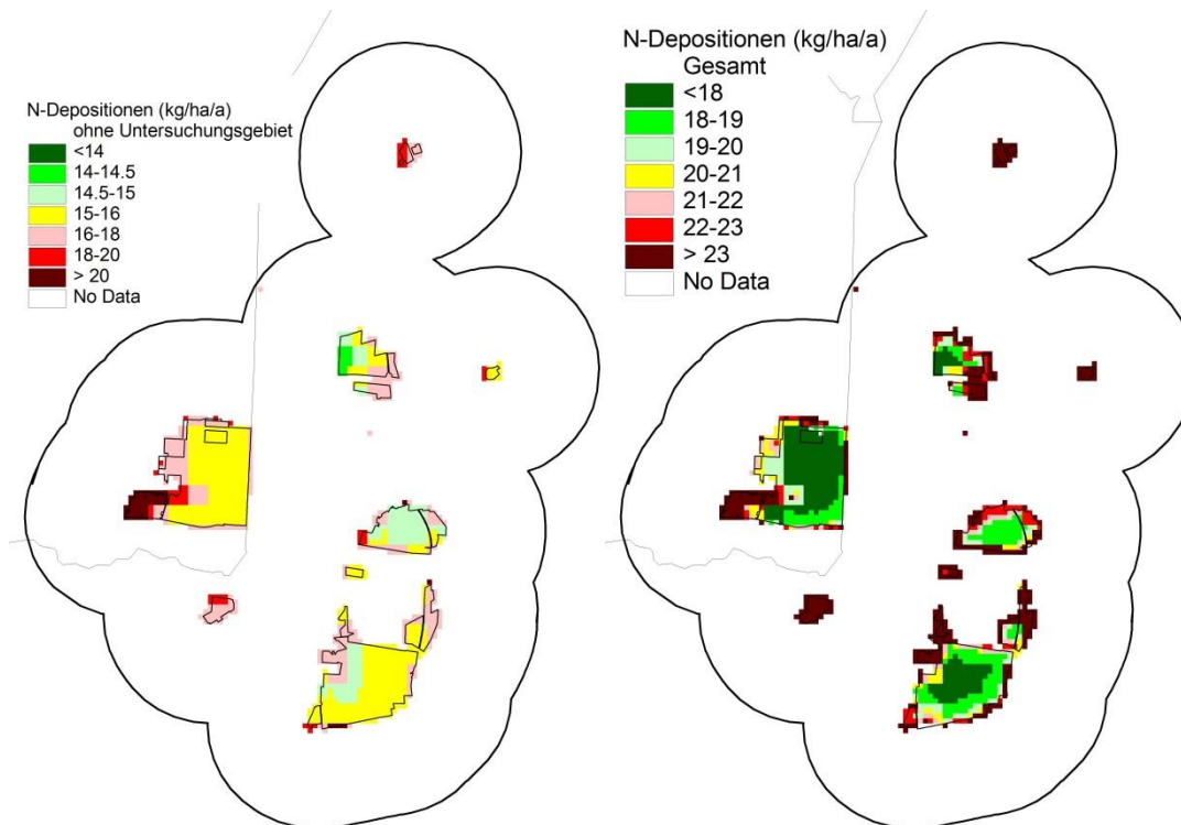
Abbildung 5.5: Berechnete Gesamt-N-Depositionen ( \text{NH}_x + \text{NO}_y ) von allen Quellen (rechts) sowie die N-Depositionen ohne Berücksichtigung der landwirtschaftlichen Emissionen im Untersuchungsgebiet (links). Angaben in \text{kg ha}^{-1} \text{a}^{-1} .
