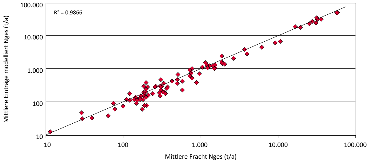
Abbildung 38: Vergleich der modellierten Stickstoffeinträge in die Vorfluter aus diffusen und punktförmigen Eintragsquellen mit gemessenen Stickstofffrachten unter Berücksichtigung der gewässerinternen Retention
