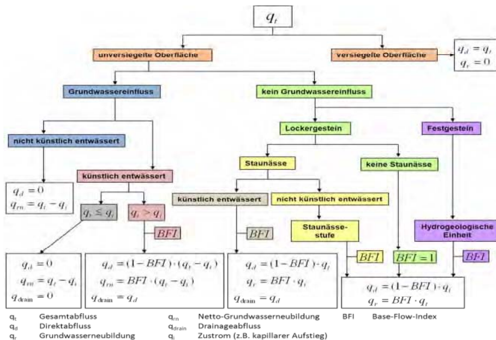
Abbildung 6: Hierarchie der abflussrelevanten Gebietseigenschaften zur Ableitung der BFI-Werte im GROWA-Modell
