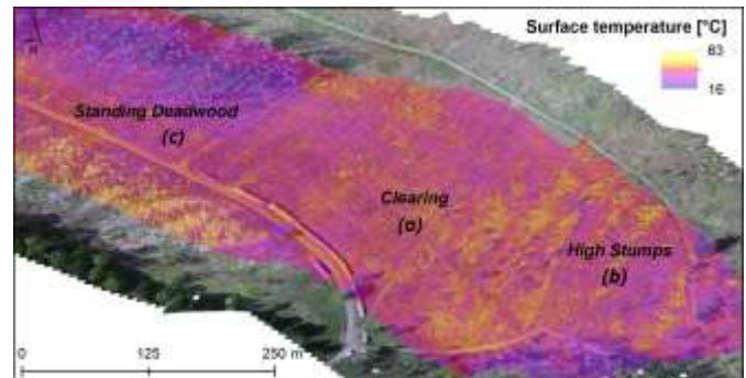
© B. Putzenlechner: Orthophoto im optischen Spektralbereich und Landoberflächentemperatur aus UAV-Befliegung (Flughöhe von 100 m) in der Region Südharz mit unterschiedlichen Varianten forstlichen Managements: (a) Räumung, (b) Hochstubben und (c) Dürrständer
