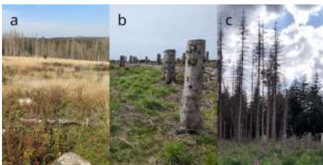
© B. Putzenlechner, S. Grieger: Varianten forstlichen Managements gestörter Fichtenflächen: (a) Räumung, (b) Hochstubben (abgestorbene Fichten, auf eine Höhe von 2 bis 4 m gekürzt) und (c) Dürreständerinseln (teilweise geräumte Inseln mit einer schachbrettartigen Anordnung noch stehender, abgestorbener Fichten)
