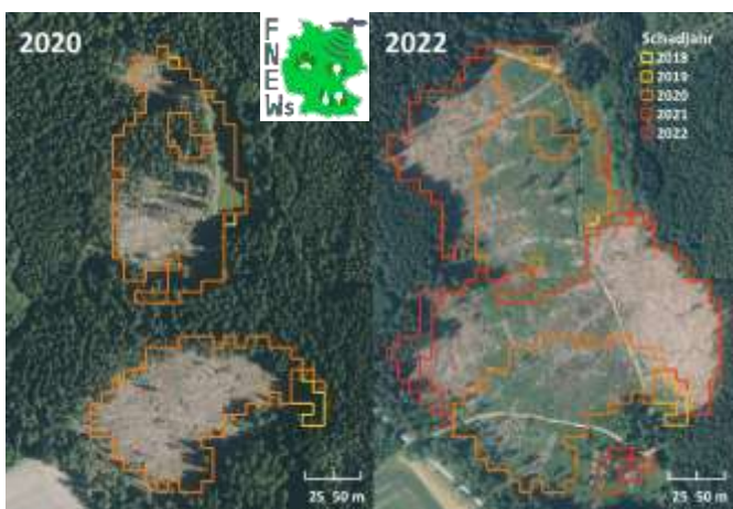
© Thünen-Institut: Erkannte Schadflächen des FNEWS-Jahresproduktes. Hintergrund: Luftbilder (© GeoSN) aus den Jahren 2020 (links) und 2022 (rechts)
